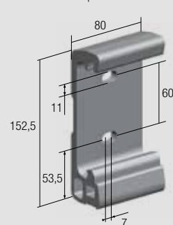
Wand-plafond montage
