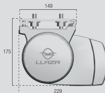
Plafondbevestiging
