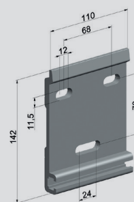
Muurconsole
