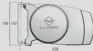
Muurbevestiging
