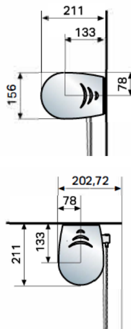
Afmetingen van de steunen
