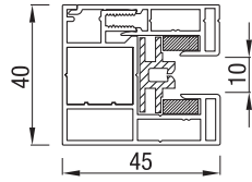
SMART TWEDELIJGE GELEIDER
