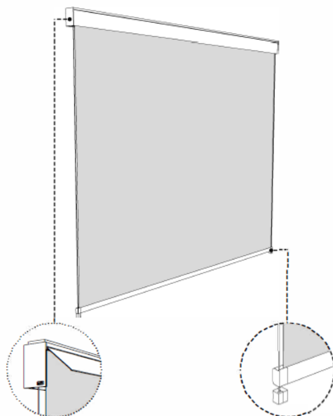
Screen met kast en kabelgeleiding, optioneel met Led-verlichting
